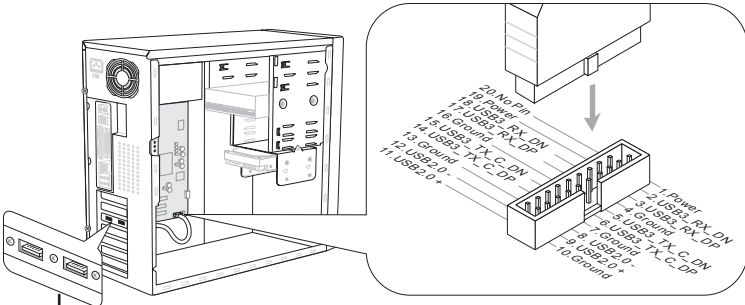
USB 3.0 브래킷 (옵션)
