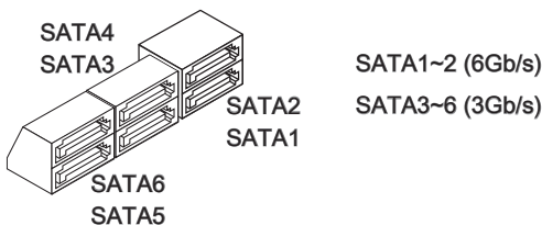
* MBレイアウト参照図
