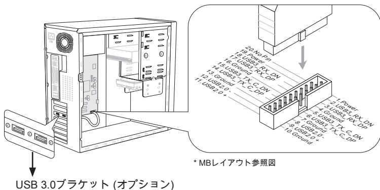
USB 3.0ブラケット (オプション)
