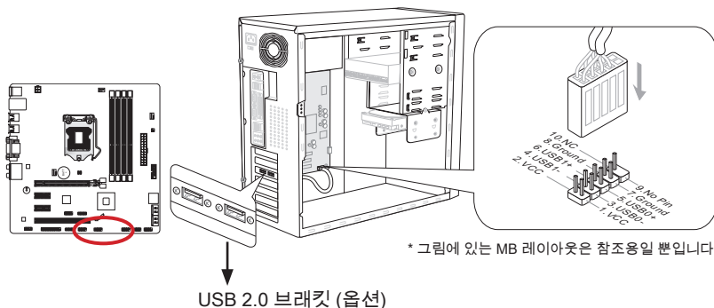
USB 2.0 브래킷 (옵션)
