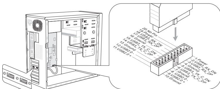
USB 3.0 转接口 (选配)
